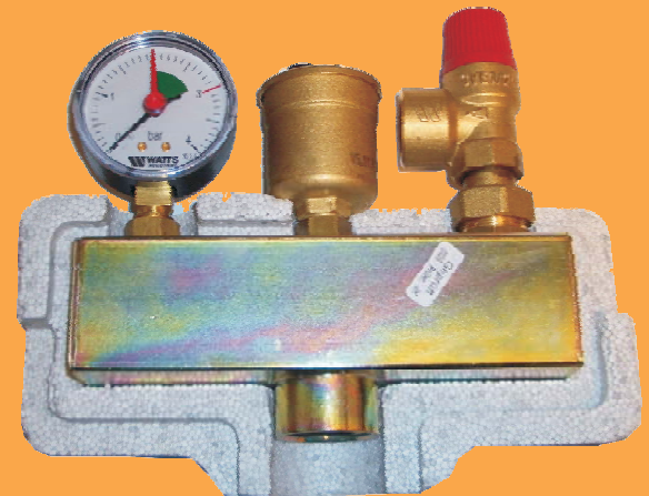
Kesselanschluss / Sicherheitsgruppe inkl. Schnellentlüfter Sicherheitsventil und Barometer
